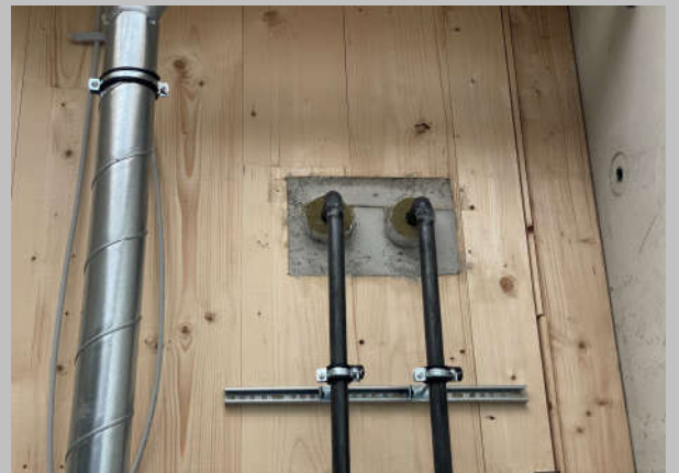
Brandschutzgerechte Heizungsrohrdurchführung Decke, (Nasseinbau)
